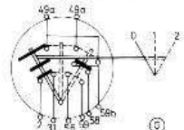
Schaltbild Zünd-Lichtschalter
